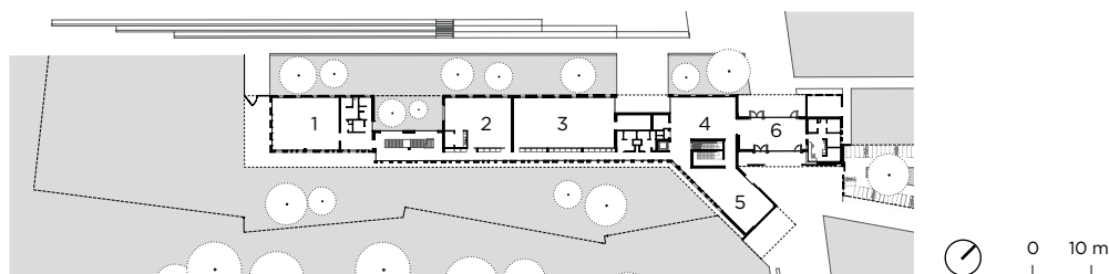
Plan de rez-de-chaussée du bâtiment d'accueil
