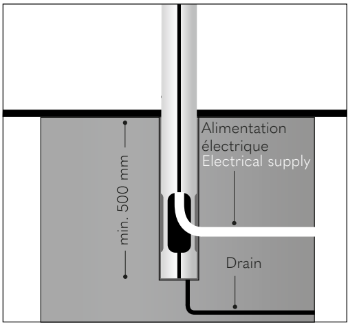
Variante avec mât enterré Variation with burried pole
